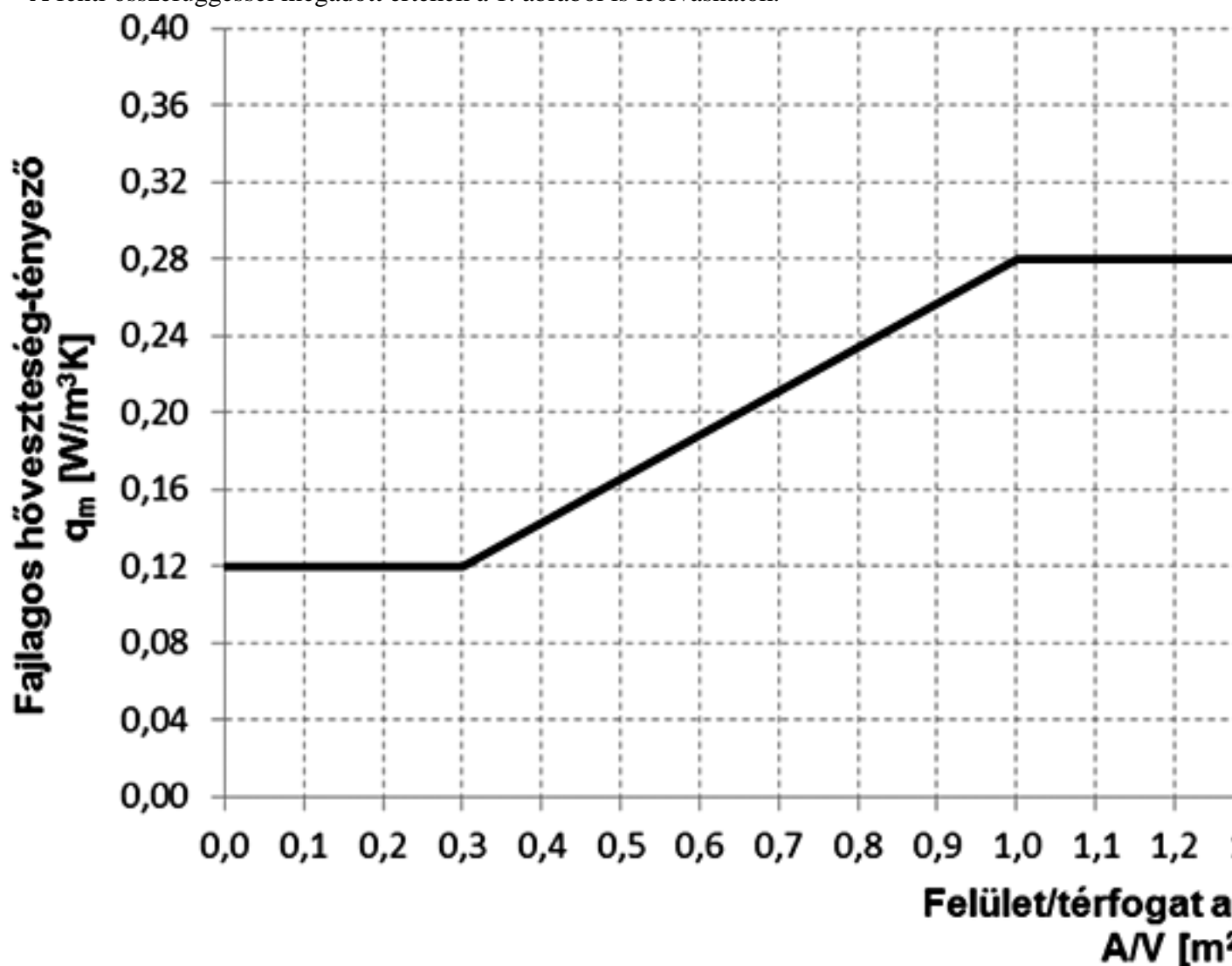
1. ábra: A fajlagos hővesztés-tényező követelményértéke.
