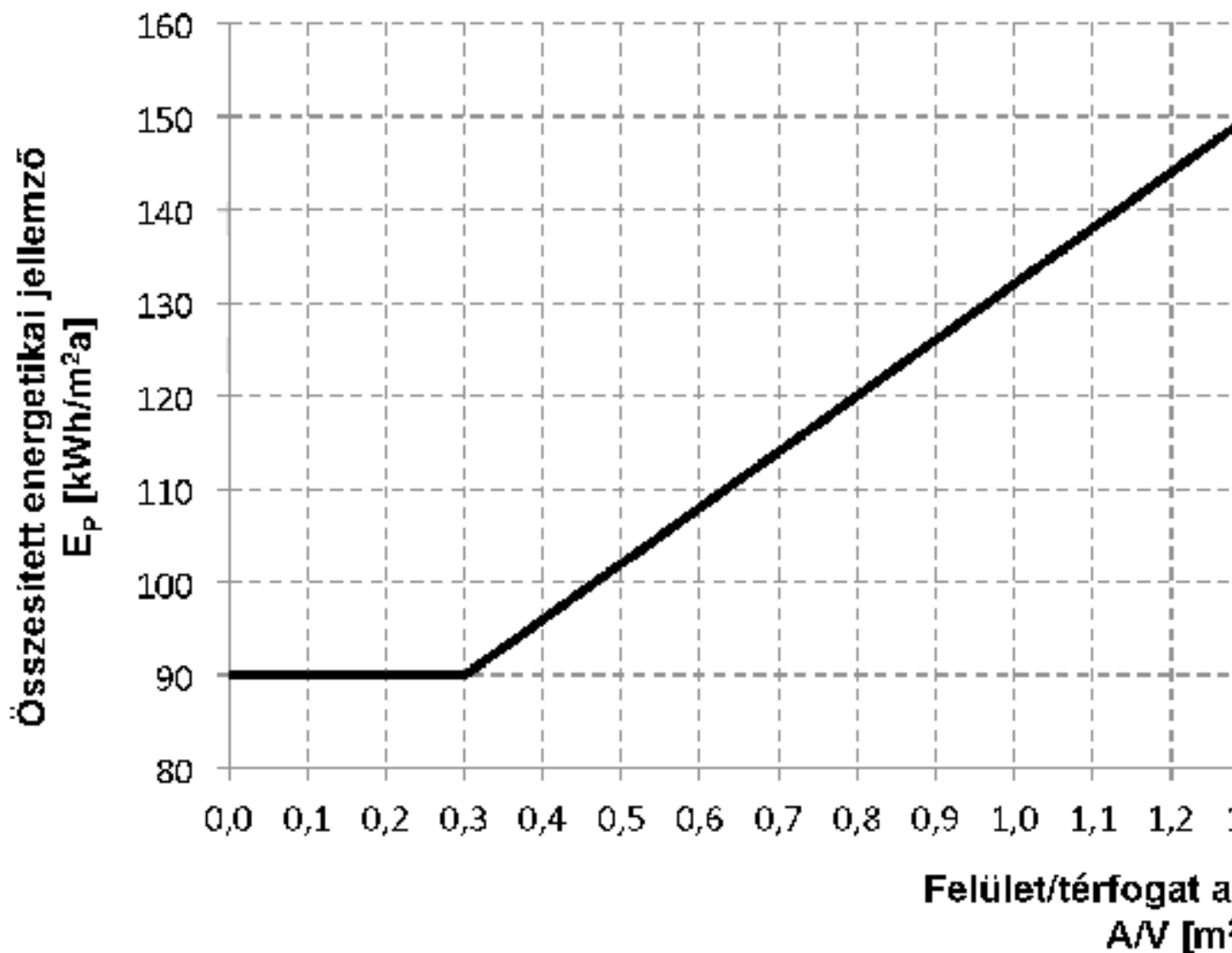
1. ábra: Oktatási épületek összesített energetikai jellemzőjének követelményértéke (világítási energia igényt is beleértve)
