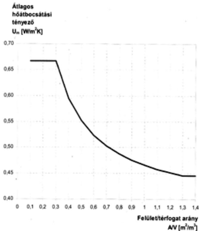
2. ábra: Az átlagos hőátbocsátási tényező követelményértékei
