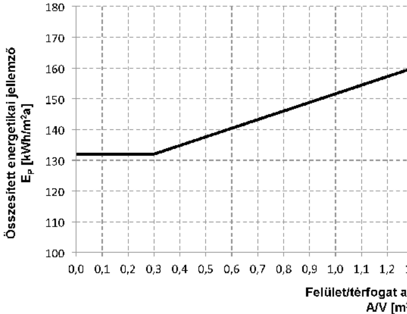
1. ábra. Irodaépületek összesített energetikai jellemzőjének követelményértéke (a világítási energia igényt is beleértve)
